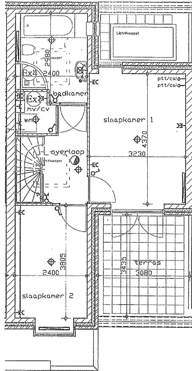
1e verdieping
