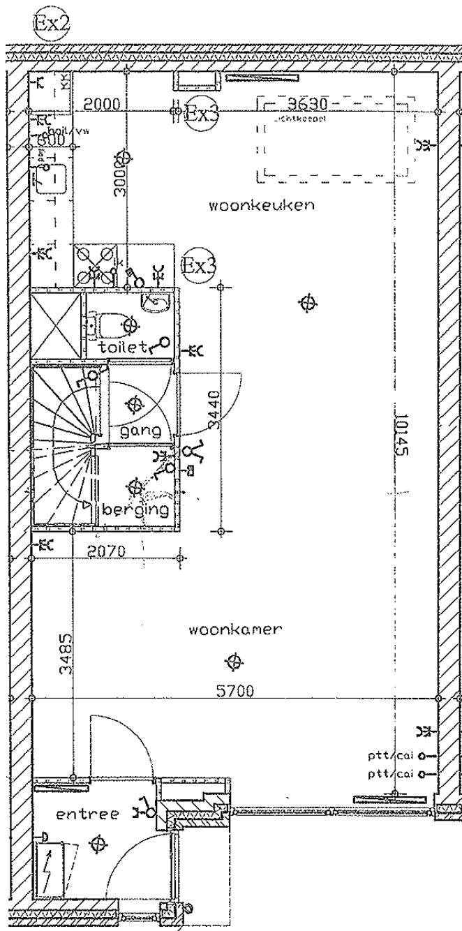
Begane grond
